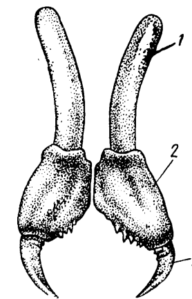
Рис. 26. Ядовитый аппарат тарантула (по П. И. Мариковскому, 1958):
