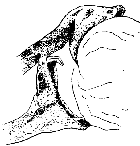
Рис. 76. Механизм укуса змей (по Карру, 1977)
