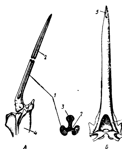
Рис. 57. Схема строения колючки спинного плавника некоторых активно-ядовитых рыб (по Холстеду, 1970):
