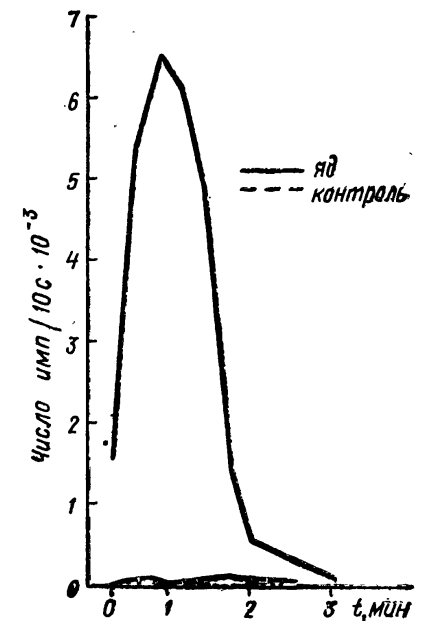
Рис. 27. Влияние яда паука Loxosceles reclusa (0,5 мкг/мл) на спонтанную активность вентральной нервной цепочки таракана Periplaneta americana (по Фоилу и соавт., 1979)
