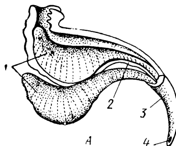
Рис. 20. Ядовитый аппарат скорпионов (по Физали, 1922):
