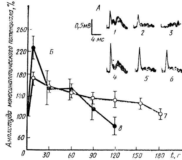
Рис. 84. Влияние яда среднеазиатской кобры Naja oxiana (0,5 мг/кг) на рефлекторную передачу в спинном мозге кошки (по Орлову, Гелашвили, 1975):
